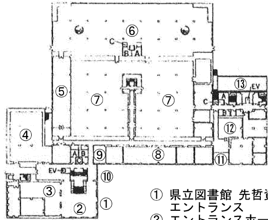
1F平面図
