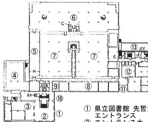
1F平面図
